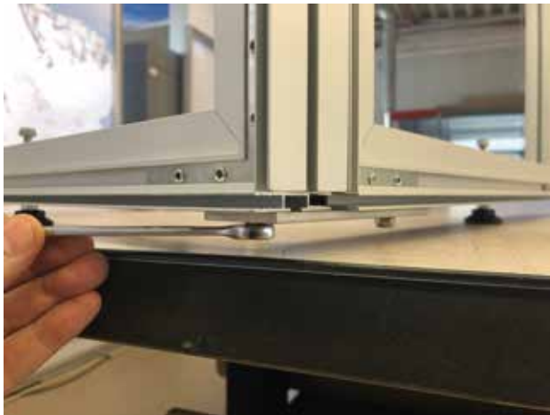
5. Stumpfe-Stossverbindung unten
