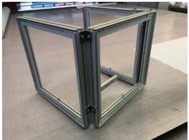
4. 90° Rahmenverbindung
