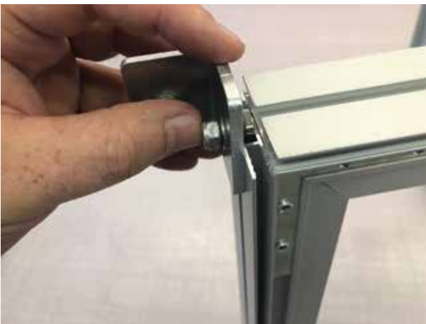
3. 90° Rahmenverbinder
